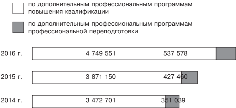
Рисунок 1. Статистика ДПО
